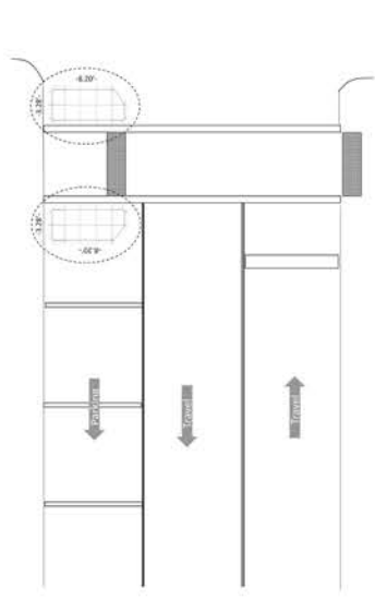
Pedestrian Curb Extension (Bulb-out)
